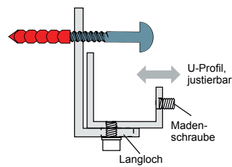
unteres Befestigungselement
