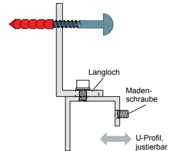
oberes Befestigungselement
